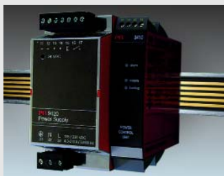
9400 Силовая шина DIN для монтажа и питания модулей серии 9000. Возможно подключить до 27 модулей.
