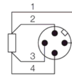
Схема подключения
