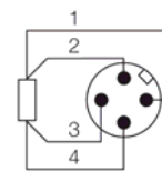
Схема подключения
