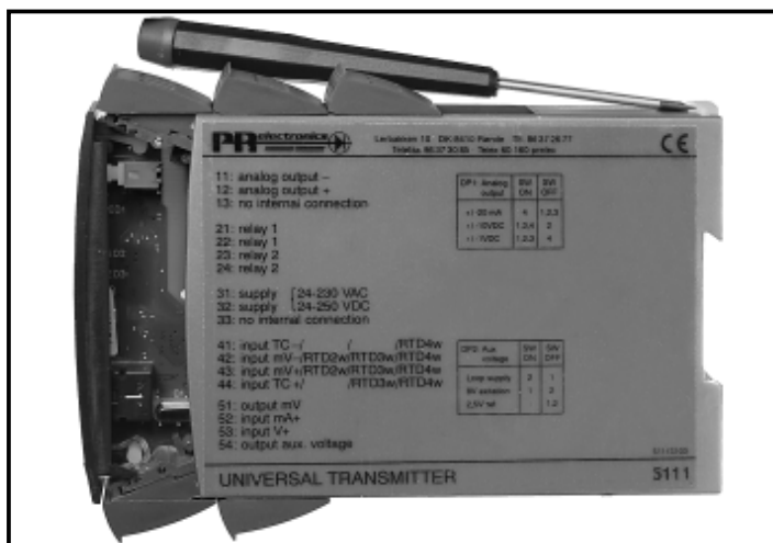
Илл. 2: Так вынимают печатную плату.
