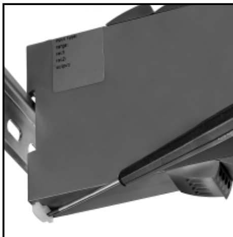
Илл. 1: Отсоединение от рейки DIN
