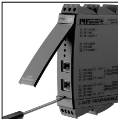
Илл. 3: Контакт программирования.
