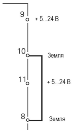
2 разных источника положит. напряжения с общей землей
