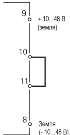
Последовательная схема, + или (-) 10...48 В
