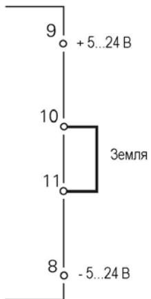
Последовательная схема, двуполярное питание (+ / -)
